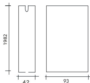
Skyvedørparti Standardhøyde 2000 mm
