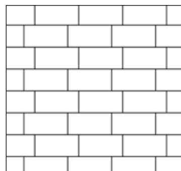
KVARTSTENSFORBANDT
